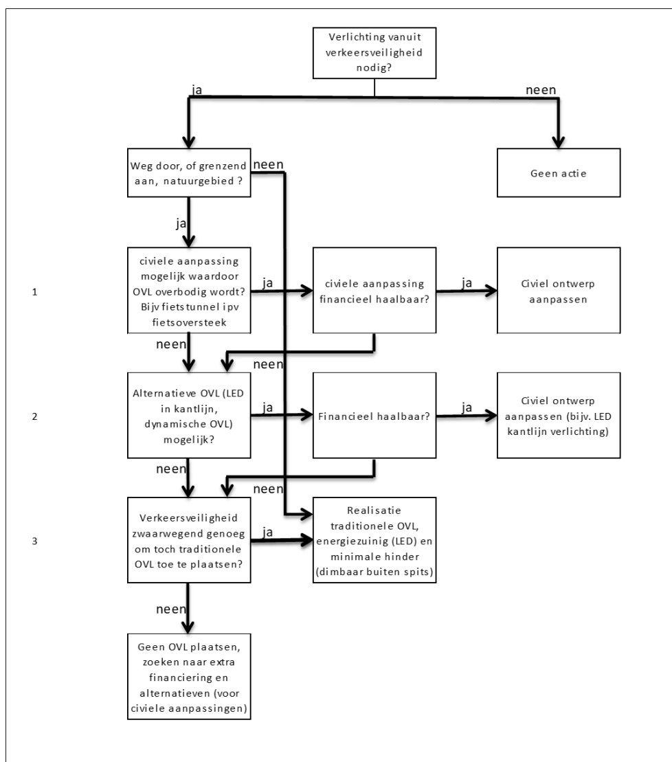
Figuur 1: Stappenplan plaatsen openbare verlichting.
