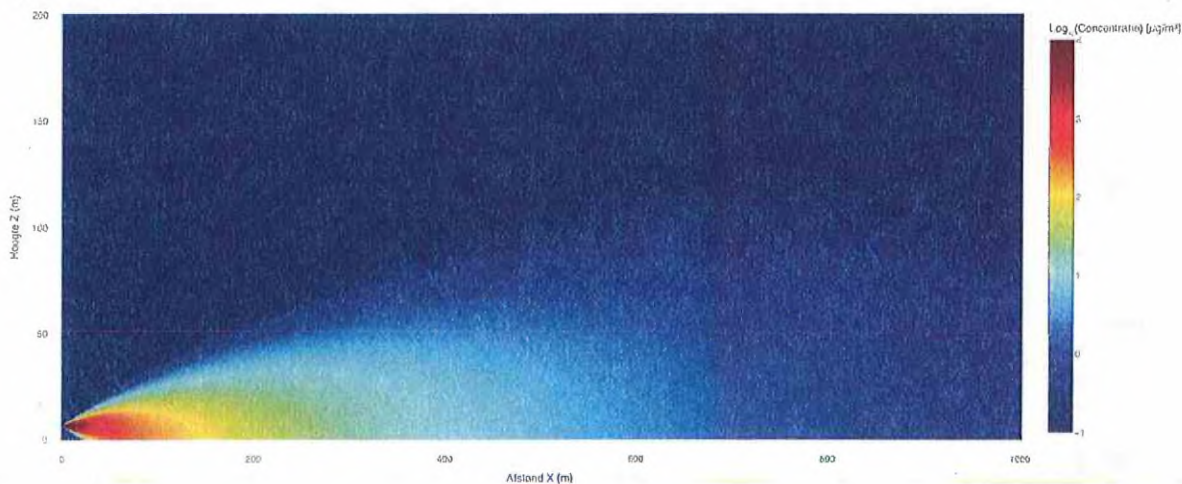
Concentratie in X-Z vlak (Y=0m) Gaussian Plume met Depositie
