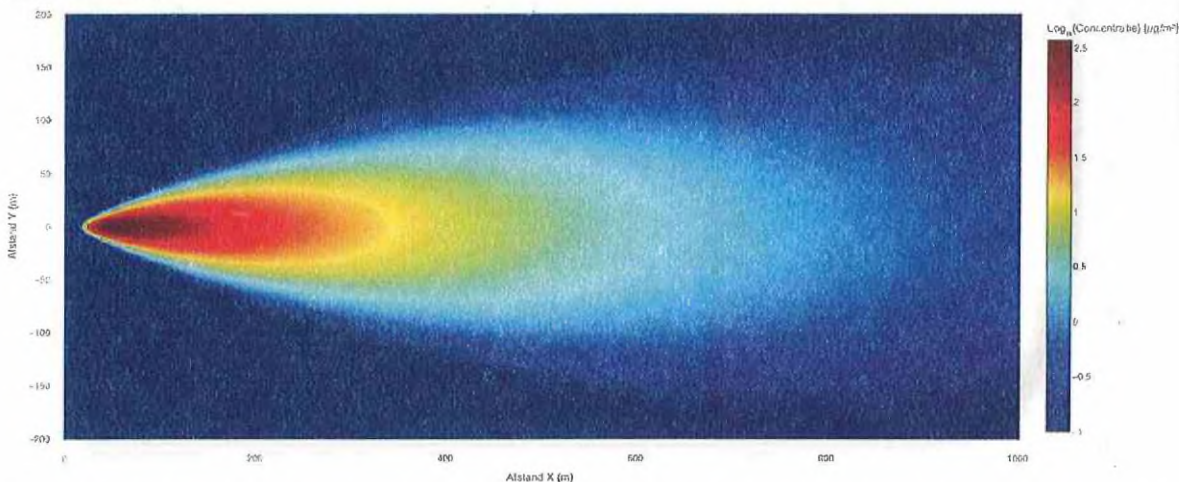
Figuur 5: Berekende concentratie in het X-Y en X-Z vlak benedenwinds. De concentratie staat op een logaritmische schaal (log-10), duidelijk is dat enkele duizenden meters effect van de stal niet meer aanwezig is.
