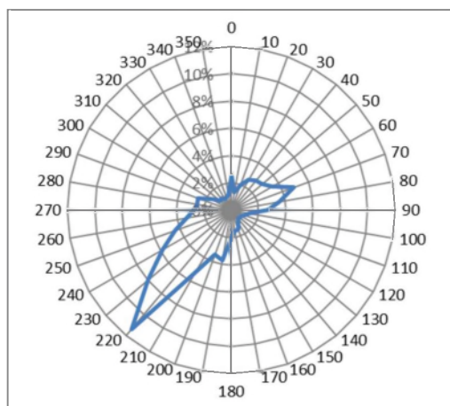
Figuur 1. Frequentiewindroos 2023
