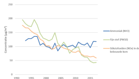
Figuur 6. Ontwikkeling concentraties ammoniak, fijn stof (PM10) en NOx (NOx: concentraties in de bebouwde kom) 1990-2017 14
