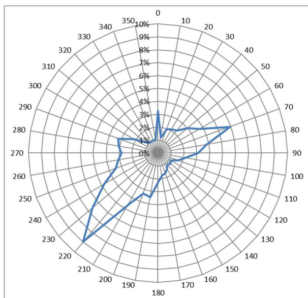
Figuur 3: Frequentieverdeling (%) van de windrichting (2022)
