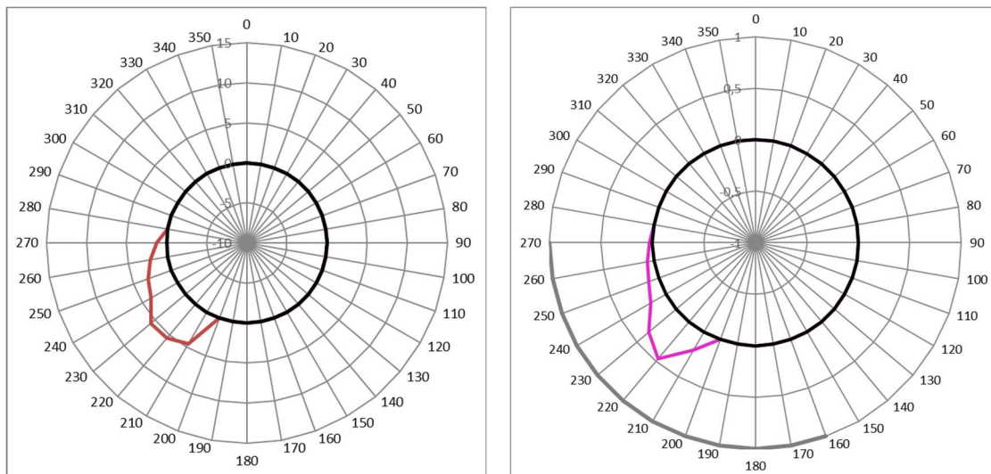
Figuur 7: Links: windroos van het NO 2 concentratieverschil (µg/m 3 ) tussen locatie Ossendrecht en Doel in 2022.
