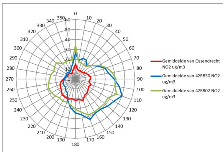
Figuur 6 : Concentratiewindrozen van NO 2 (µg/m 3 ) op locatie Ossendrecht, Borgerhout (42R802) en Doel (42R830) in 2022.
