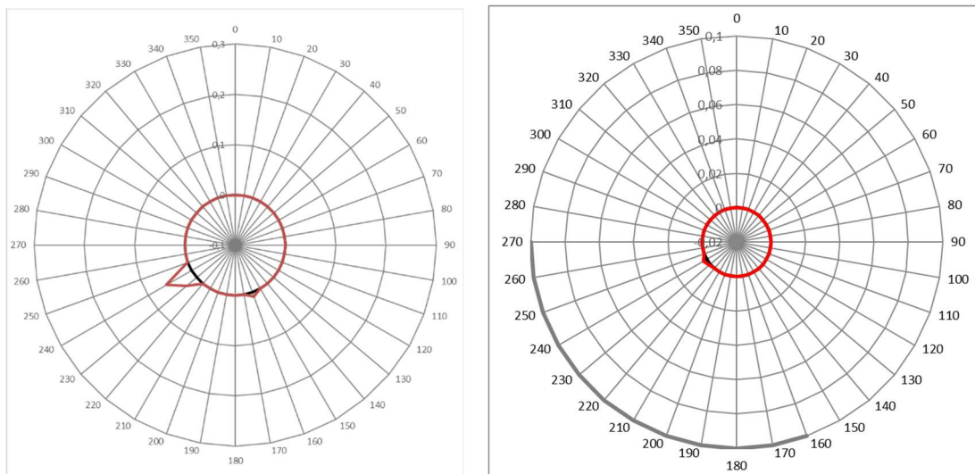
Figuur 9: Links: windroos van het benzeenconcentratieverschil ( \mu\text{g}/\text{m}^3 ) tussen locatie Ossendrecht en de achtergrondconcentratie van 0,6 \mu\text{g}/\text{m}^3 in 2022. Rechts: windroos van de bijdrage ( \mu\text{g}/\text{m}^3 ) per sector op locatie Ossendrecht.
