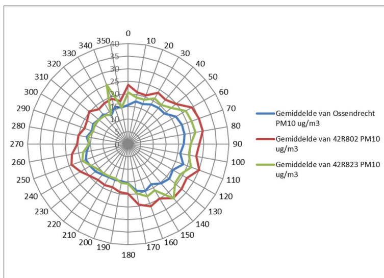
Figuur 4 : Concentratiewindrozen van PM 10 (µg/m 3 ) op locatie Ossendrecht, Borgerhout en Beveren in 2022.
