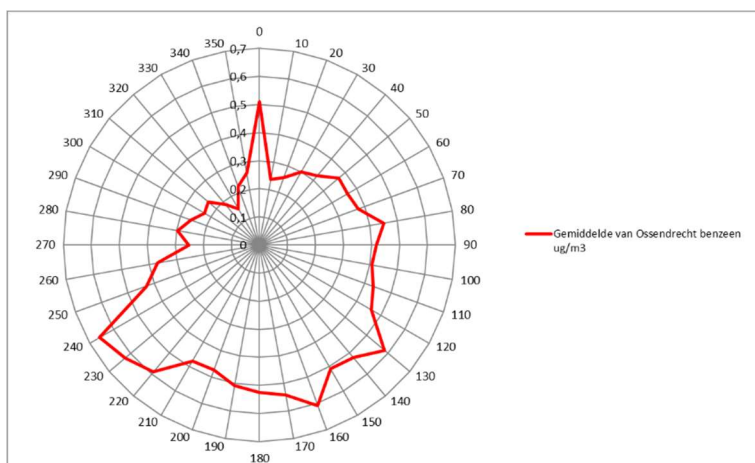
Figuur 8: Concentratiewindroos van benzeen (µg/m 3 ) op locatie Ossendrecht in 2022.
